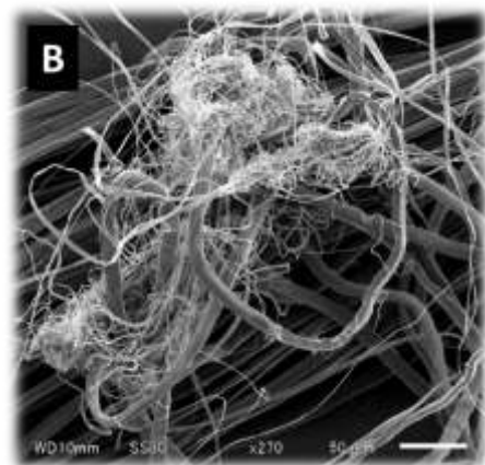
図2. アルカリ処理後に離れた繭糸分離細繊維 (点線枠付近: 矢印はフィブロイン)
